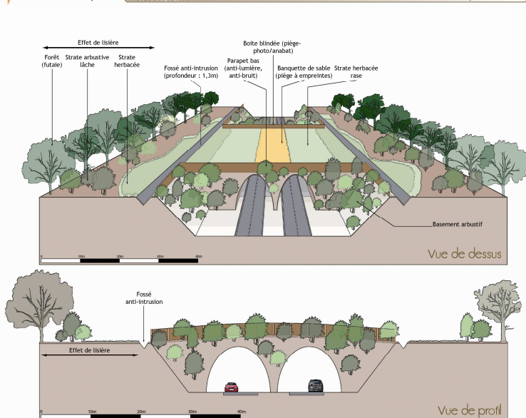
biotope Schéma d'aménagement d'un passage à grande faune Pont Buse - Etat projeté Source : Biotope 2011
